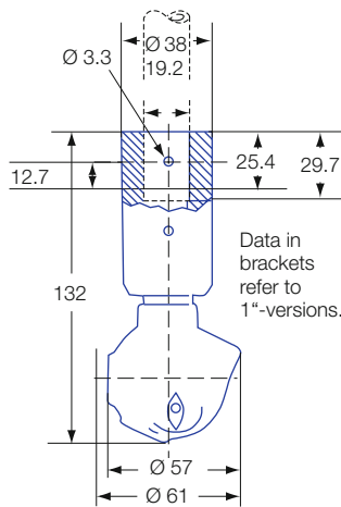
Slip-on connection ASME - BPE 1997 (OD-Tube)
