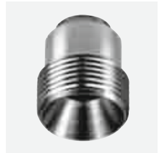
Welding nipple 092. 020. 17. 00. 04 Material: AISI 316Ti
